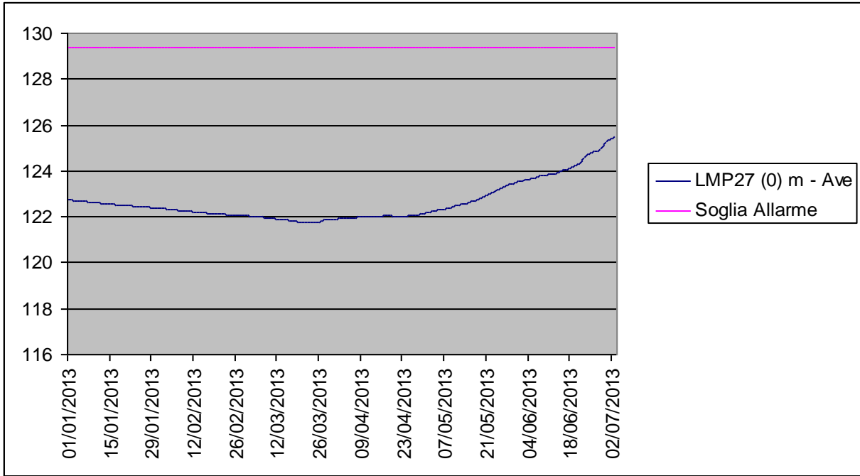
Pozzo 27 (Livelli di falda)
