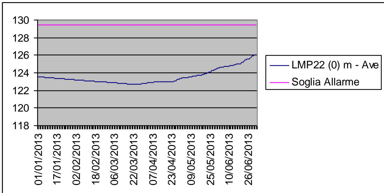
Pozzo 22 (Livelli falda)
